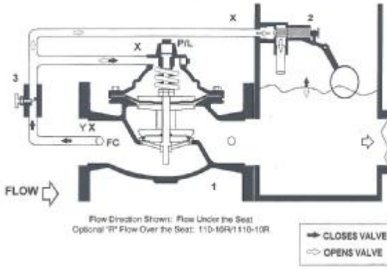
WATTS ACV-110-10 定水位閥 (維持固定液位)
