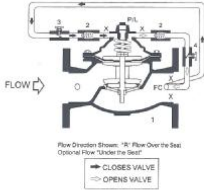
WATTS ACV-118-3 可調啓/閉速度逆止閥
