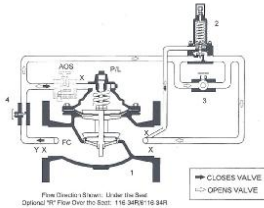
WATTS ACV-116-34 手動復歸低壓關斷閥
