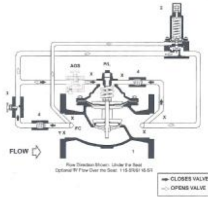
WATTS ACV-116-5 逆止持壓閥
