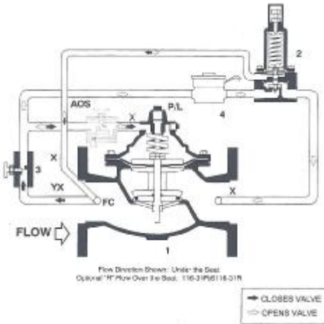
WATTS ACV-116-31 電磁持壓閥
